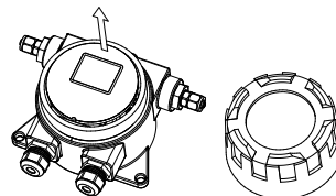
②往上取下亚克力板
