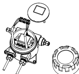
⑤把线束接到端子上
